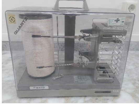
SATO marka, NS II-Q model nem ve sıcaklık ölçüm ve kayıt cihazı.
